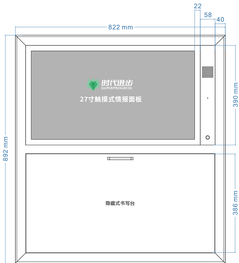
正视图
